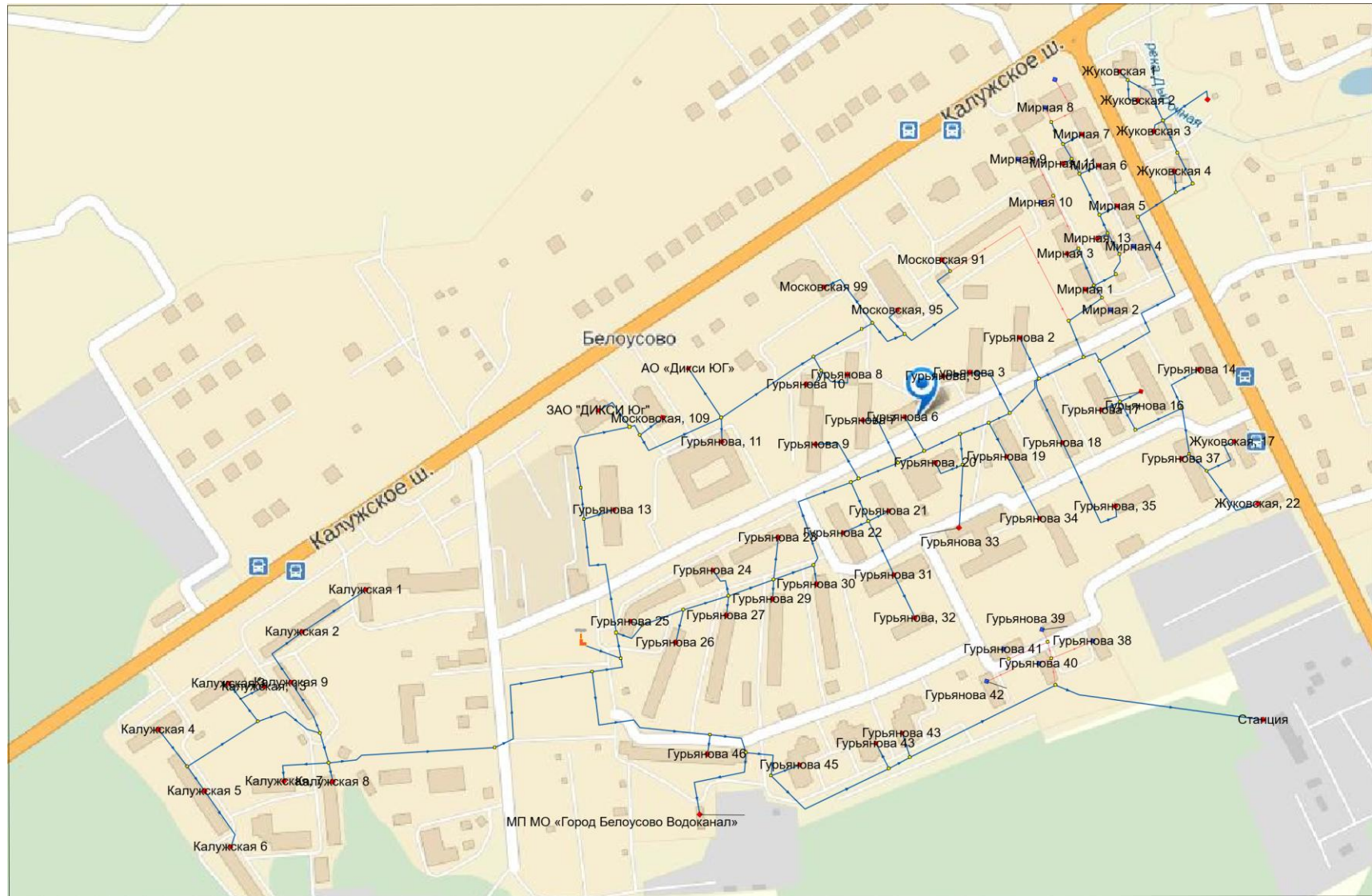
Рисунок 2 - Схема тепловых сетей котельной по ул. Гурьянова, 25/1
