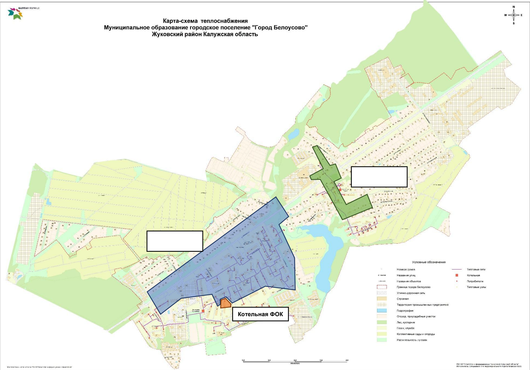
Рисунок 1 - Зоны деятельности котельных МУП «Теплоснабжение»
